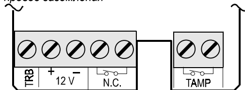
Рисунок 6. Клеммная колодка детектора GlassTech
