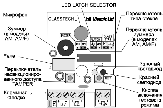
Рисунок 5. Схема печатной платы
