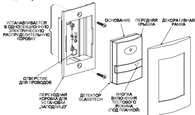
Рисунок 3. Детекторы GlassTech-F и –AM/F. КОНСТРУКЦИЯ И СБОРКА.
