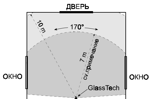
Рисунок 1. Пример зоны действия детектора
