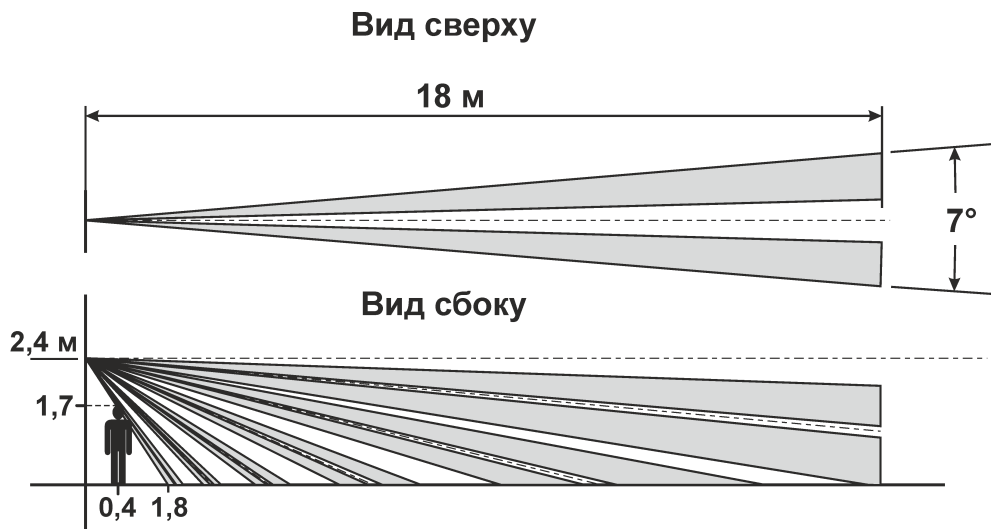
Рисунок А.2 – Диаграмма направленности извещателя ИНС-101 Штора
