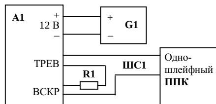
Рис.1 Схема подключения извещателя с объединенной передачей извещений “Тревога” и “Вскрытие”
