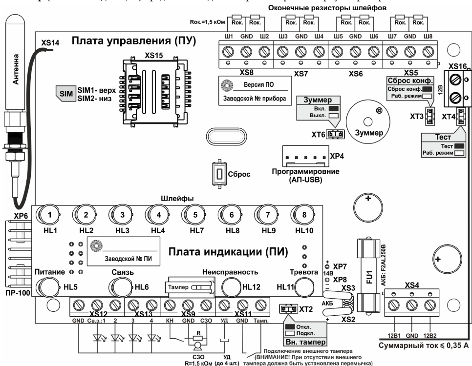
Рисунок 1 - Плата управления
