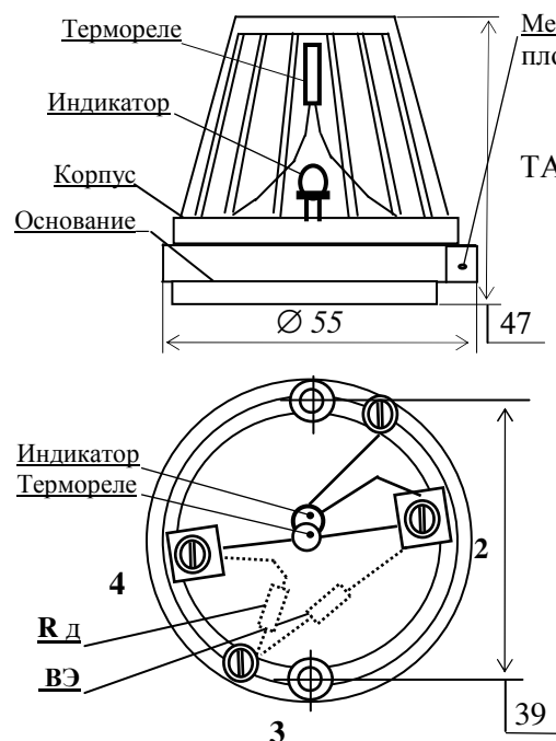
Рис. 1. Габаритные и установочные размеры, общий вид и расположение элементов в корпусе извещателя с замыкающимся контактом
