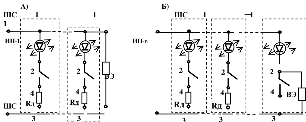
Рис. 2 Варианты включения извещателя с замыкающимся контактом в шлейф сигнализации приемно-контрольного прибора:
